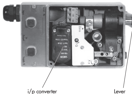
Fig. 3: Type 4763 Positioner
